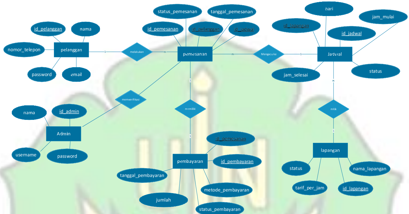
Gambar 4. ERD Sistem
