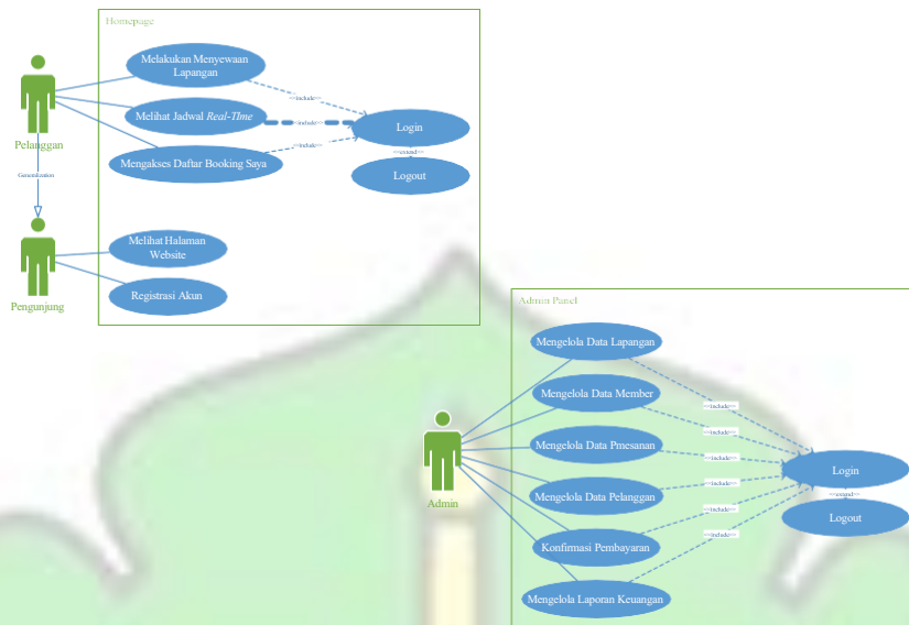
Gambar 2. Use Case Diagram Sistem Penyewaan Lapangan Bulu Tangkis
