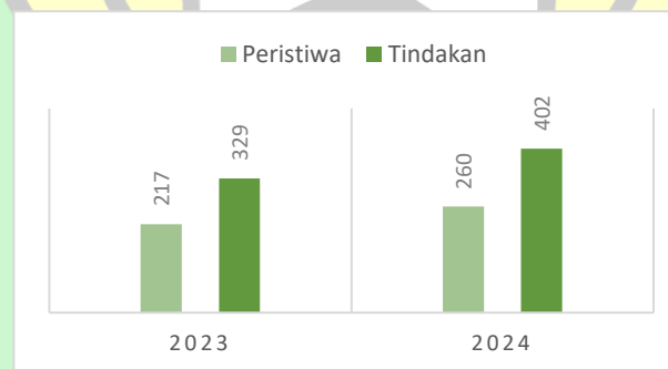
Diagram 1.1 angka pelanggaran kasus toleransi beragama
