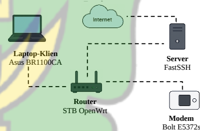
Gambar 2 Topologi Jaringan
