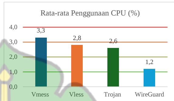
Gambar 10 Grafik Penggunaan CPU Rata-rata
