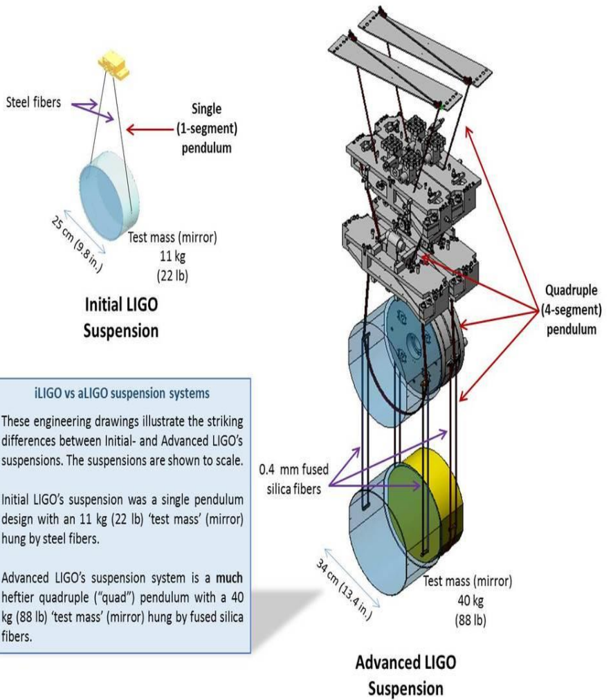
Gambar 4.13 Sistem suspensi iLIGO dan aLIGO(Sumber: LIGO)
