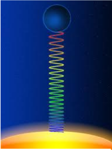
Gambar 1.12 Ilustrasi pergeseran merah gravitasi
