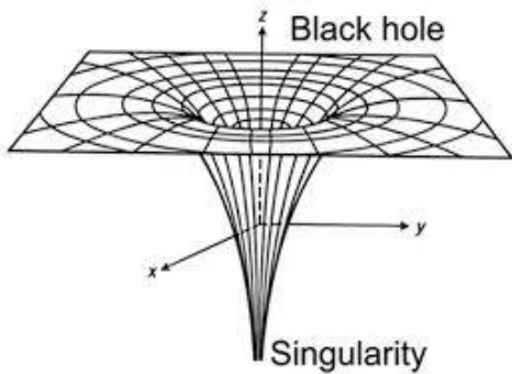
Gambar 2.1 Singularitas dan lubang hitam
