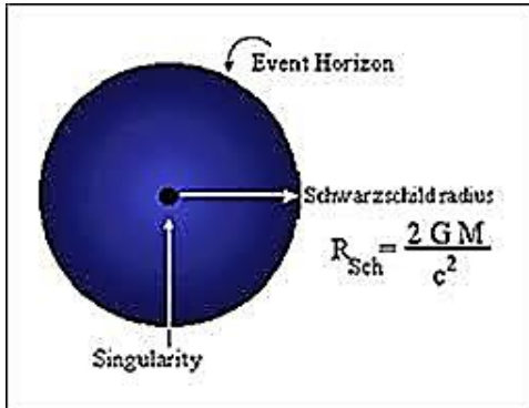
Gambar 3.1 Struktur Black Hole Schwarzschild
