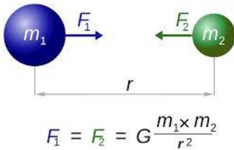
Gambar 1.8 Ilustrasi gaya gravitasi Newton
