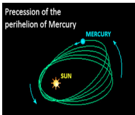
Gambar 1.11 Presisi perihilion Merkurius
