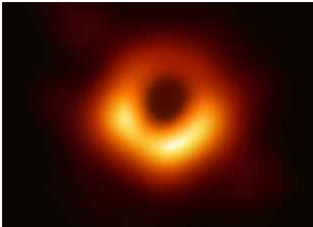
Gambar 5.2 Bayangan lubang hitam
