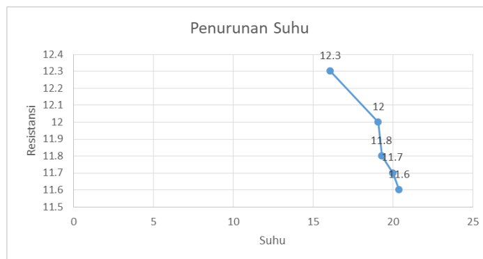
Gambar 3. Grafik Penurunan Nilai Resistansi Terhadap Suhu Pada Termistor PTC Dalam Media Dingin.
