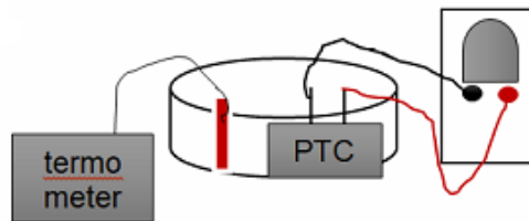
Gambar 1. Rangkaian Termistor PTC dengan Termometer dalam media dingin.
