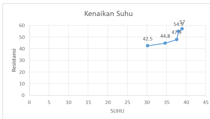
Gambar 4. Grafik Kenaikan Nilai Resistansi Terhadap Suhu Pada Termistor PTC Dalam Media Panas.
