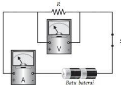
(Sumber Netya Nurachmandinan) Gambar 2.4 Pemasangan Amperemeter dan Voltmeter Pada Rangkaian
