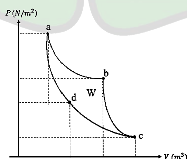
Gambar 11. Siklus mesin pemanas Carnot Sumber: Buku Fisika Peminatan untuk SMA/MA
