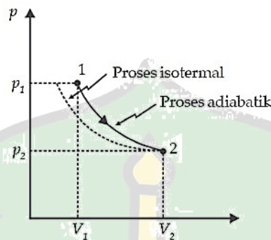
Gambar 10. Grafik Proses Adiabatik Sumber: http://fisikazone.com/proses-termodinamika/
