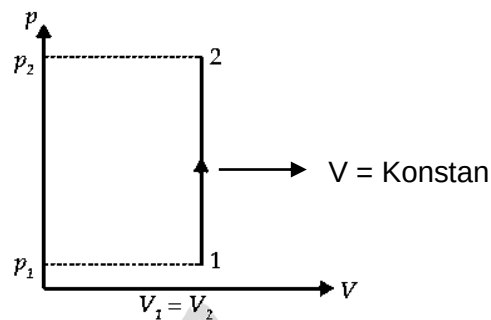
Gambar 8. Grafik Proses Isokhorik
