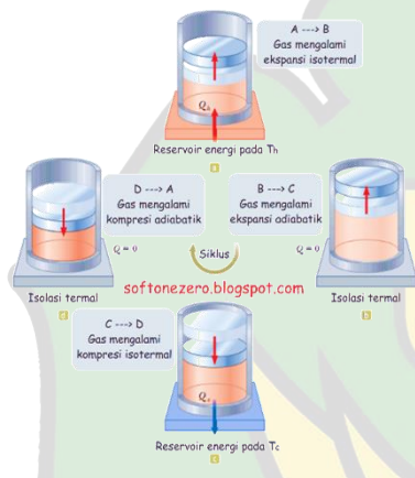
Gambar 14. Siklus Carnot, Huruf A, B, C dan D mengacu pada keadaan dari gas yang ditunjukkan pada Gambar 15 Sumber: http://softonezero.blogspot.com
