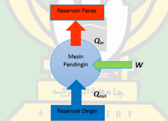
Gambar 13. Diagram aliran energi pada mesin pendingin. Mesin menyerap kalor Q_2 , dari reservoir dingin dan menyerap usaha mekanik W dari luar untuk mengalirkan kalor sebanyak Q_1 ke reservoir panas Ilustrator: Widya An Nisa Mukramah
