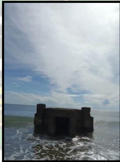
Gambar 3. 8. Posisi BML 7 terlihat semua bentuk ketika air laut surut, dan BML 14 terlihat dalam laut ketika air surut. kedua struktur BML sama bentuknya. Dalam BML 7 terdapat struktur yang ditandai dengan panah warna merah. BML 7 terdapat tiga lubang pengintai yaitu dari arah barat 1, timur 1, dan utara 1. Ketebalan dinding BML 7 ukuran 40 cm yang sama dengan struktur BML lainnya. Kemudian, lubang pengintai BML 14 terlihat hanya satu dari arah utara. Namun, di gambar tidak terlihat dengan jelas lubang pengintainya. (Dok. Penulis 8 Agustus 2021)
