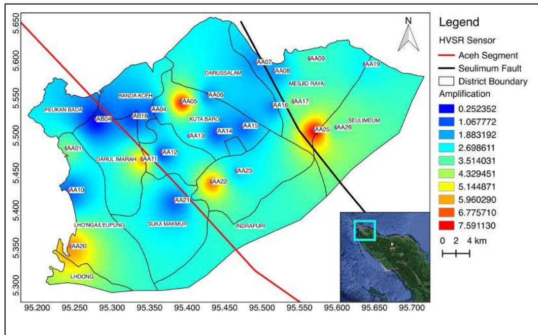
Gambar 4-5 Peta kondisi geologi Kawasan Aceh Besar berdasarkan nilai Amplifikasi tanah (tanpa topografi)
