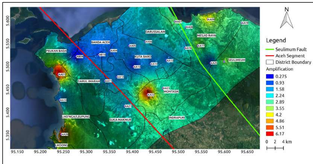
Gambar 4-4 Peta kondisi batuan kawasan Aceh Besar berdasarkan nilai amplifikasi tanah (dengan topografi)
