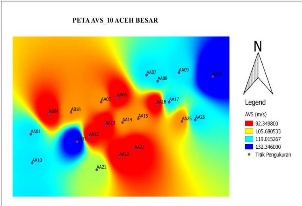
Gambar 4-9 Peta Klasifikasi Batuan/tanah Berdasarkan Kecepatan Vs (10 m)
