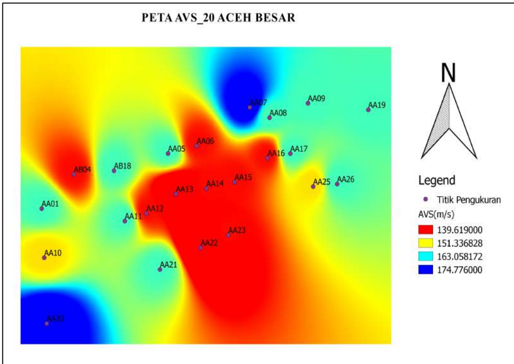
Gambar 4-10 Peta Klasifikasi Batuan/tanah Berdasarkan Kecepatan Vs (20 m)
