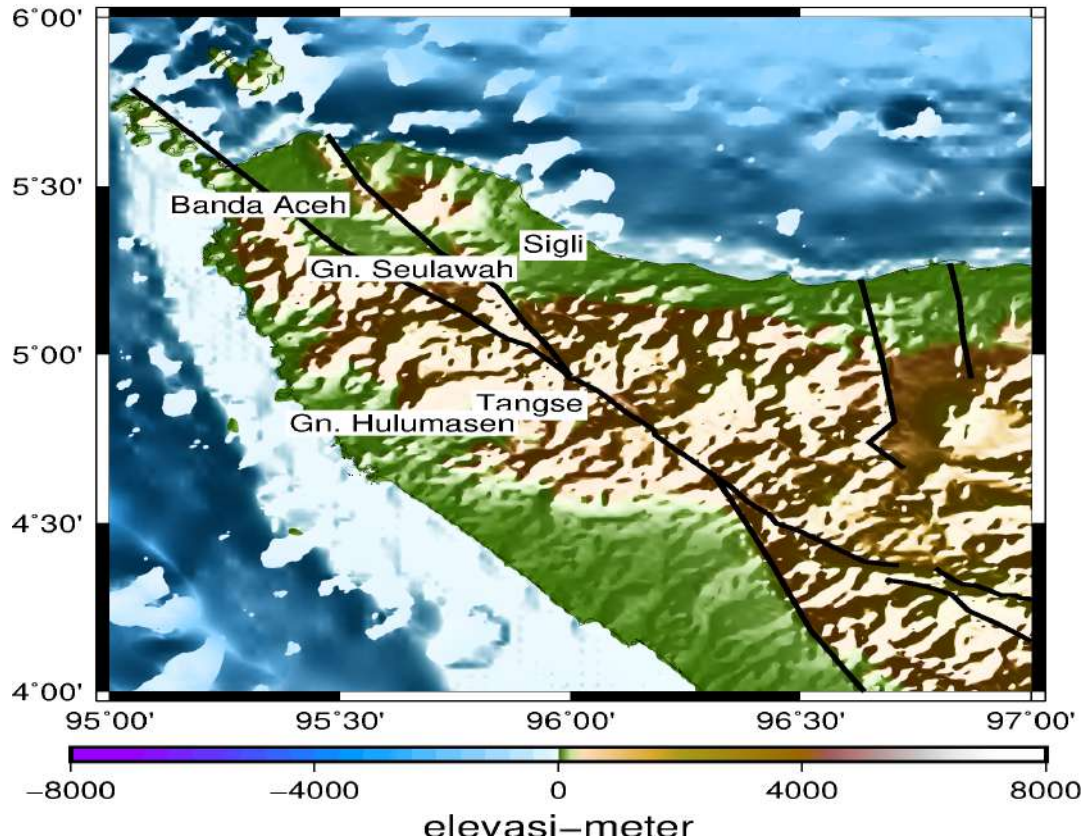
Gambar 2-4. GSF Segmen Aceh dan Segmen Seulimeum
