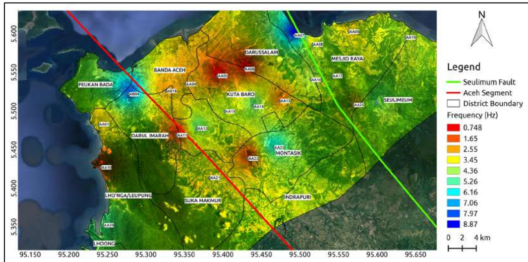
Gambar 4-2 Peta Kondisi Geologi Kawasan Aceh Besar berdasarkan nilai frekwensi dominan (dengan topografi)
