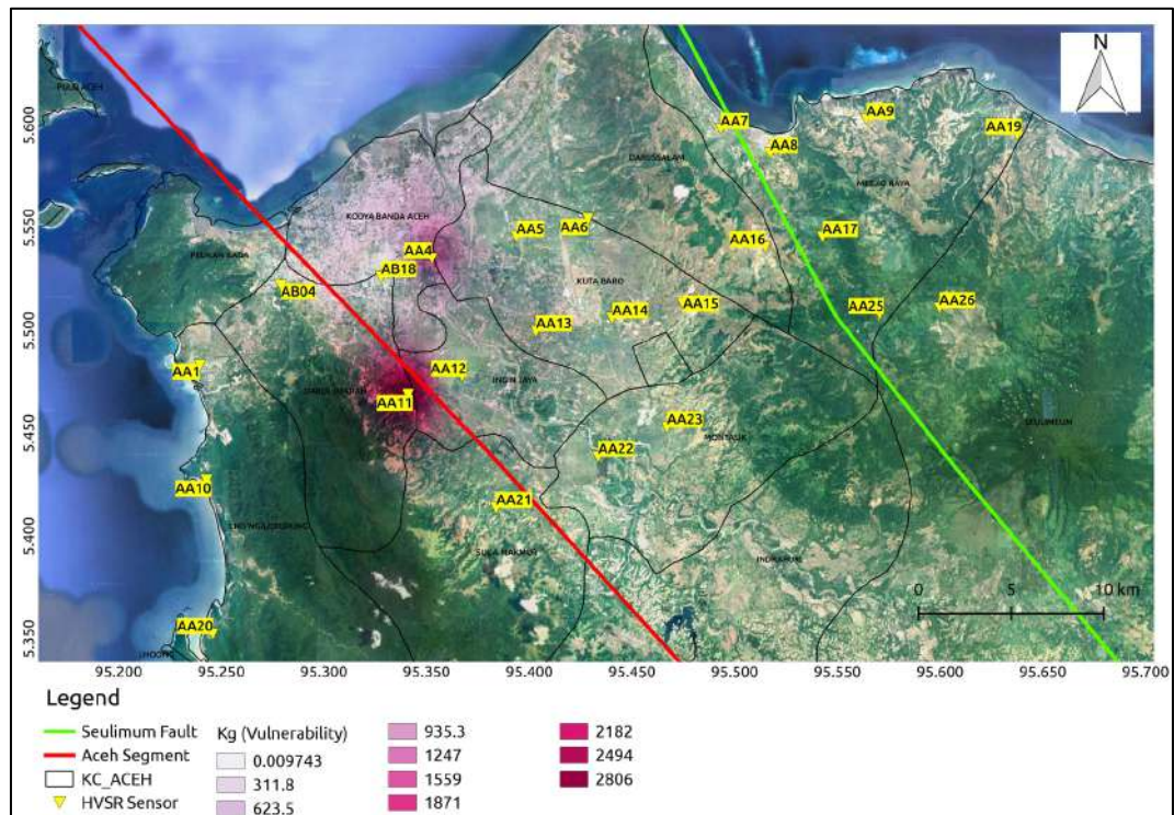
Gambar 4-6 Peta Kerentanan Seismik (Kg) Kawasan Aceh Besar
