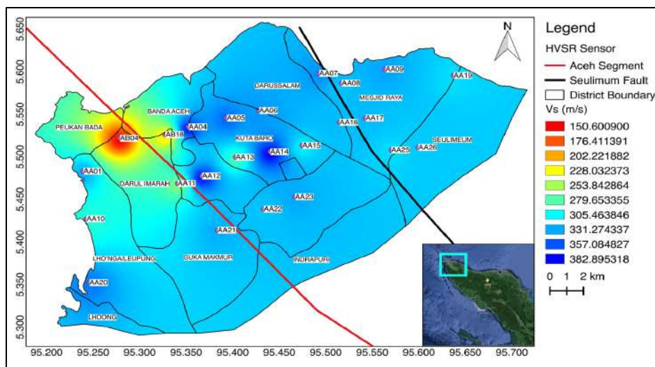
Gambar 4-7 Peta Klasifikasi Batuan Berdasarkan Data Kecepatan V_{s30}
