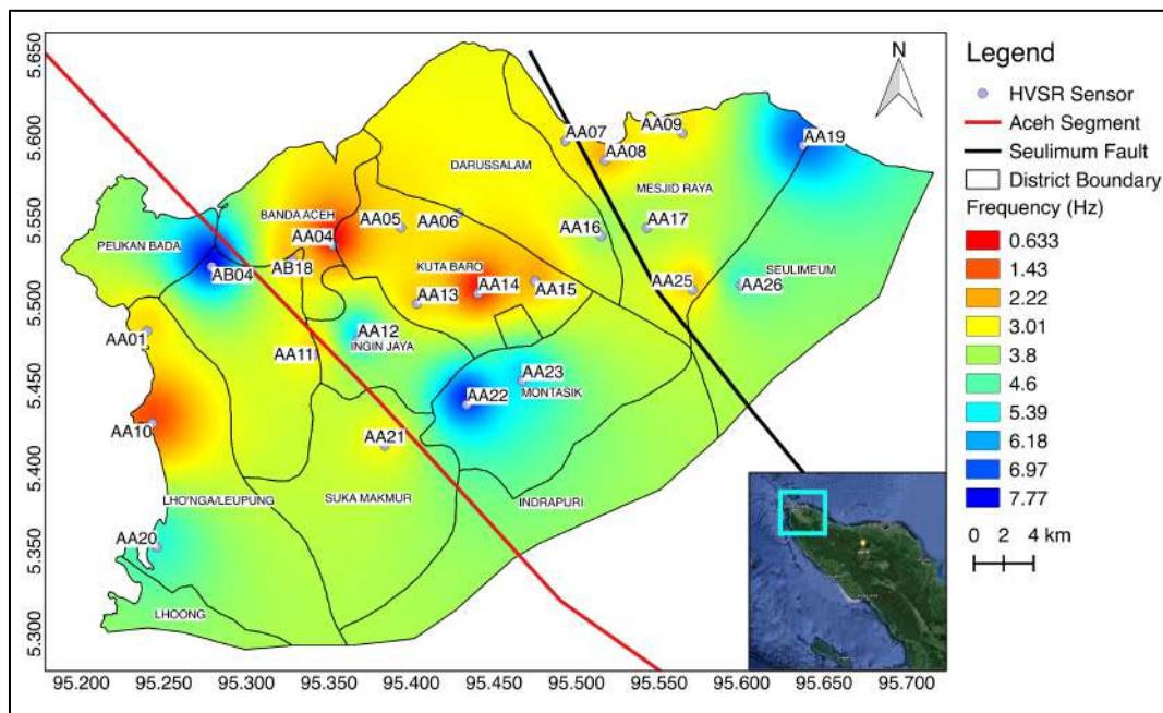
Gambar 4-3 Peta kondisi geologi Kawasan Aceh Besar berdasarkan Nilai Frekwensi Dominan (tanpa topografi)
