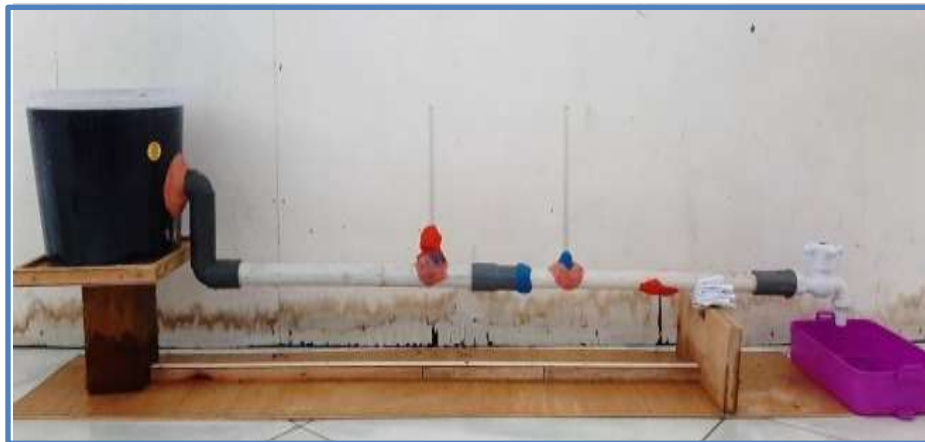
Gambar 1. Desain Percobaan Venturimeter.
