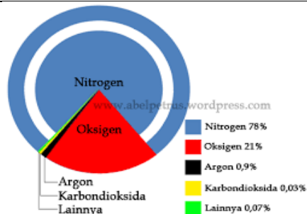
Gambar 1. Komposisi atmosfer
